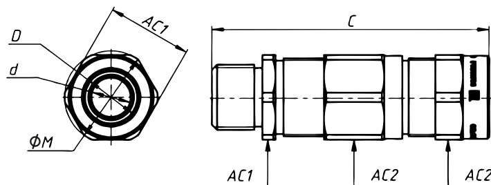
Взрывозащищенные кабельные вводы КОВ, метрическая резьба ГОСТ 24705 М
